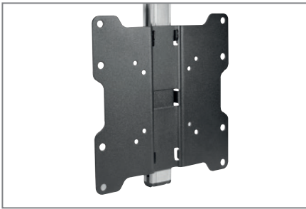
VESA min. 75 x 75 up to max. 200 x 200 mm
